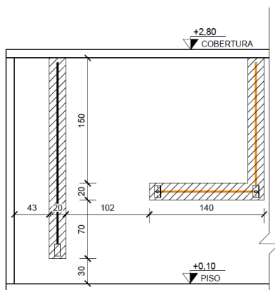
VISTA 2 - COZINHA ESC. 1 : 50
