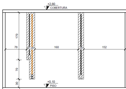
VISTA 2 - DORMITÓRIO 2
