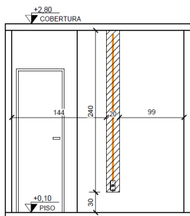
VISTA 1 - DORMITÓRIO 2
