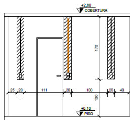
VISTA 2 - DORMITÓRIO 1
