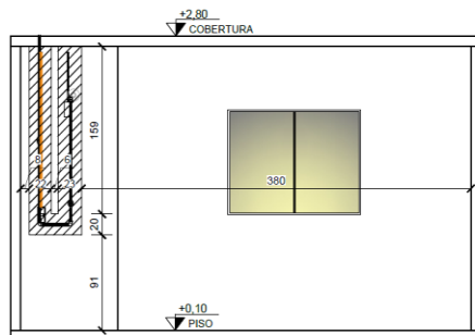
VISTA 4 - DORMITÓRIO 2
