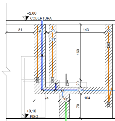
VISTA 1 - COZINHA ESC. 1 : 50
