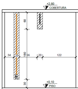
VISTA 3 - DORMITÓRIO 2
